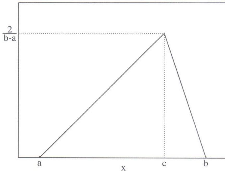
График треугольного распределения.
