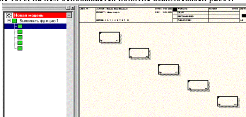
Рисунок 1.5 – Диаграмма декомпозиции
