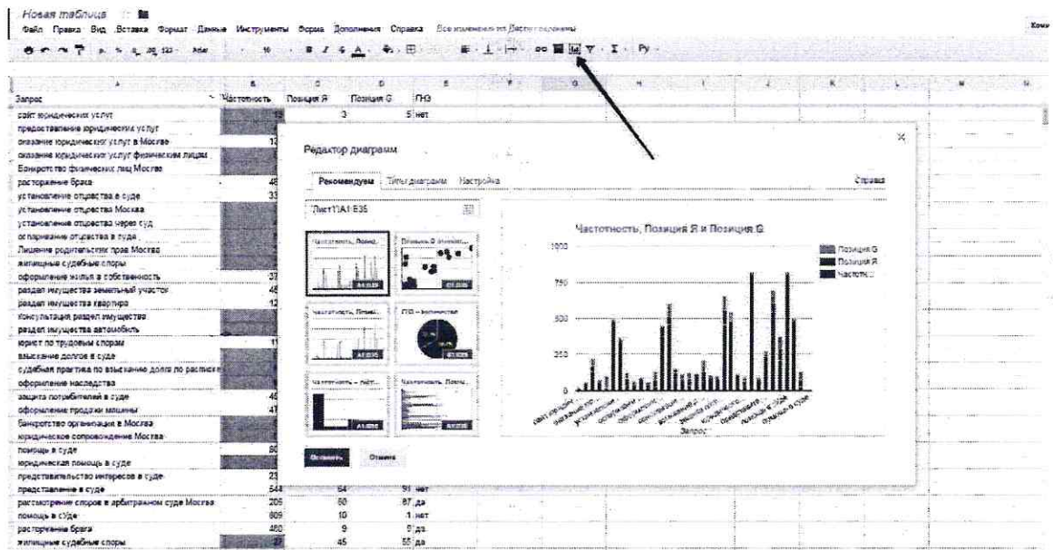
Рис.3. Google Таблица
