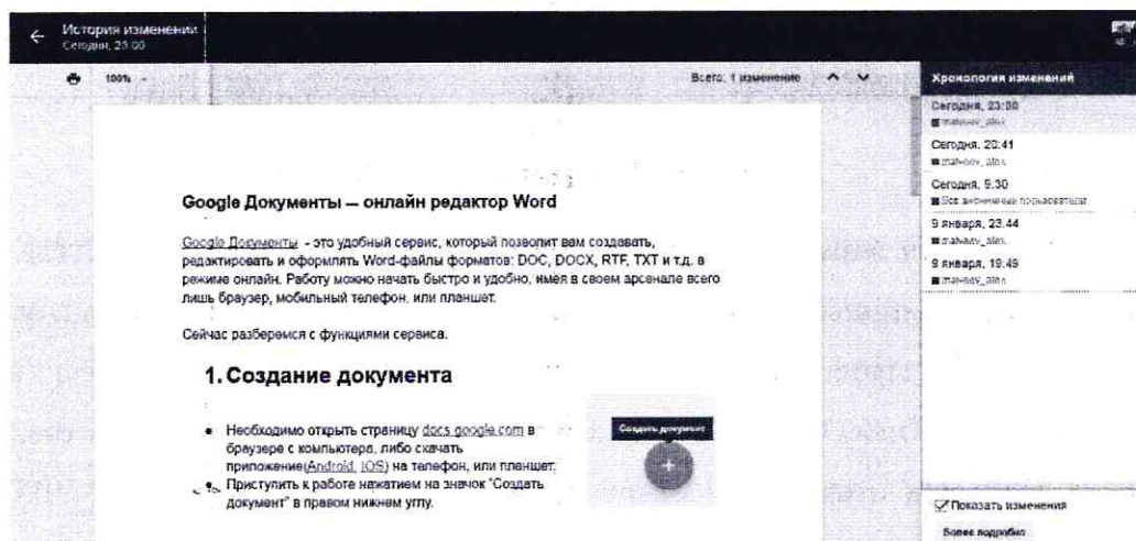
Рис.2. Google Документы
