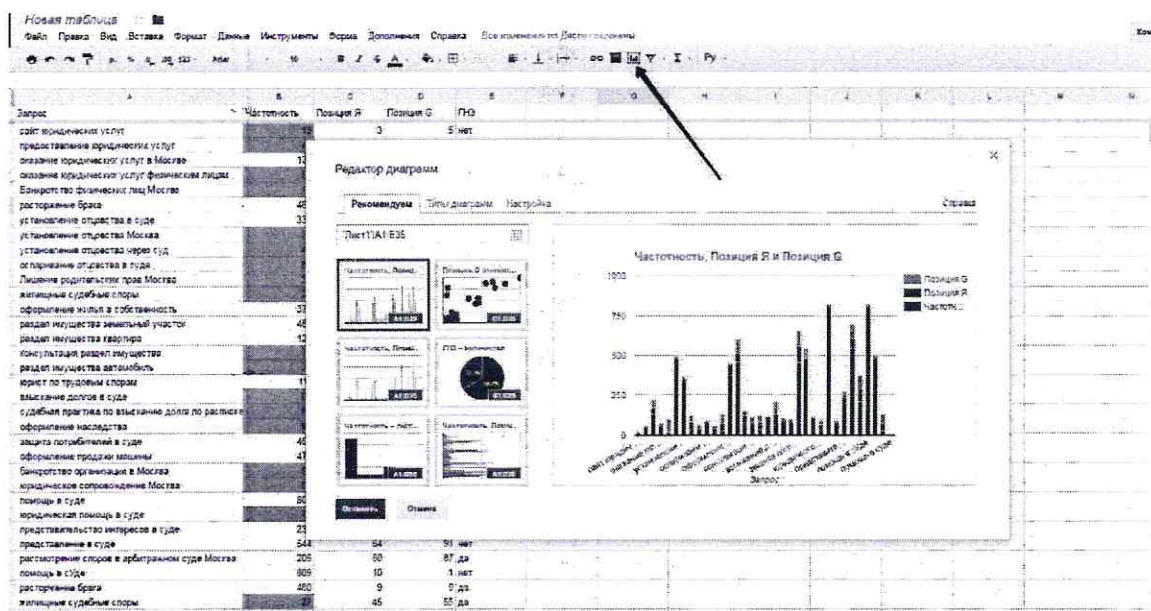
Рис.3. Google Таблица
