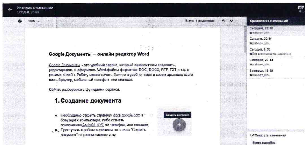
Рис.2. Google Документы
