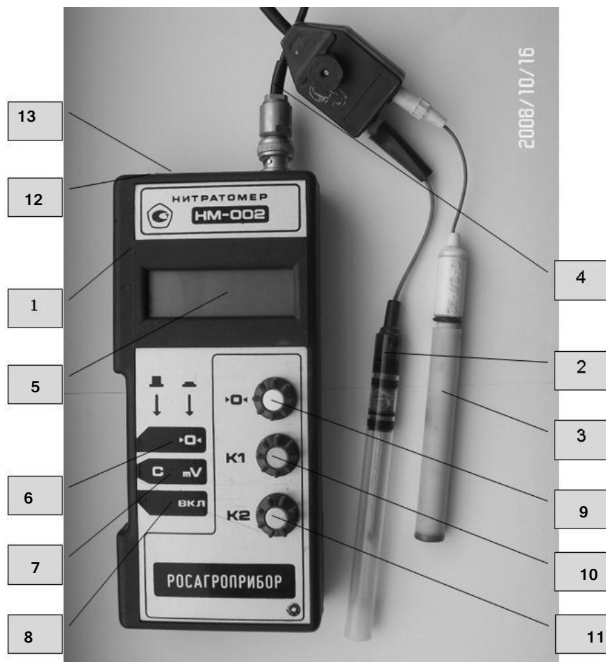
Рис. 1. Внешний вид прибора НМ 002. 1.Преобразователь. 2.Вспомогательный электрод. 8.Кнопка компенсации. 3.Измерительный электрод. 4.Соединительный кабель. 5.Индикатор. 6.Кнопка измерения приращения э.д.с. 7.Кнопка измерения концентрации и э.д.с. электродной системы. 8.Кнопка включения прибора. 9.Ручка настройки на ноль. 10 и 11. Ручки грубой и точной настройки.12. Гнездо для подключения питания 220 В. 13.Гнездо для заземления.
