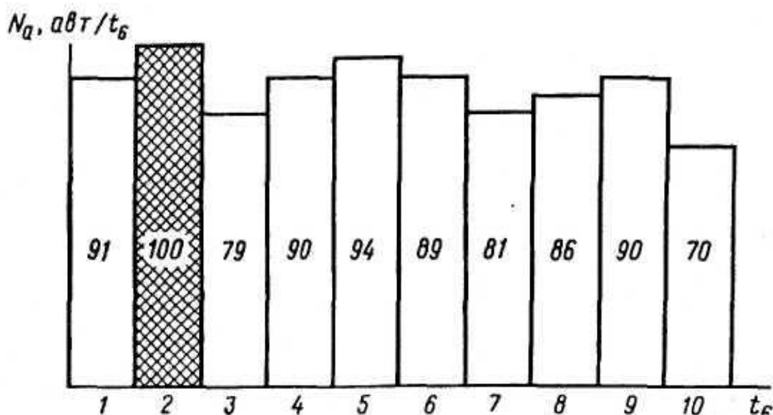
Рис. 2.5. Диаграмма интенсивности однопольного потока, полученная при определении коэффициента загрузки Z (по 6-минутным отрезкам времени)
