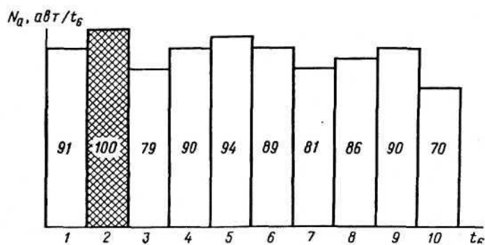
Рис. 2.9. Диаграмма интенсивности однопольного потока, полученная при определении ко-
