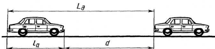
Рис. 2.4. Динамический габарит автомобиля в плотном транспортном потоке
