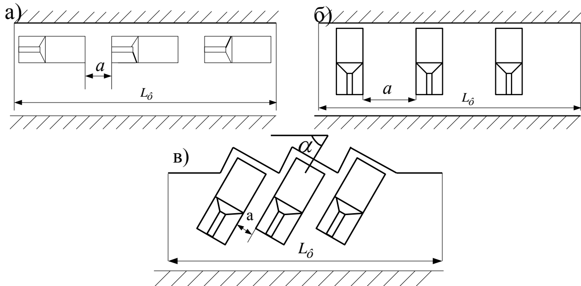
Рис. 17. Способы расстановки автомобилей при погрузке:
