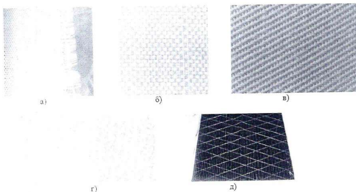
Рисунок 3 – Виды переплетения стеклотканей: а) полотняное; б) сеточное; в) саржевое; г) сатиновое; д) однонаправленная
