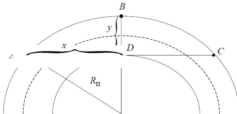
Рис. 2 – Определение величины радиуса поворота. Радиус поворота определяют по формуле
