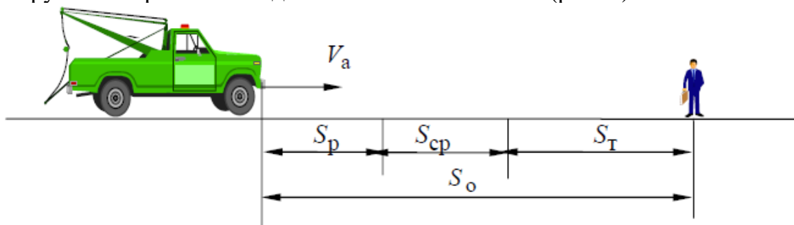
Рис. 5. – Схема для определения остановочного пути автомобиля
