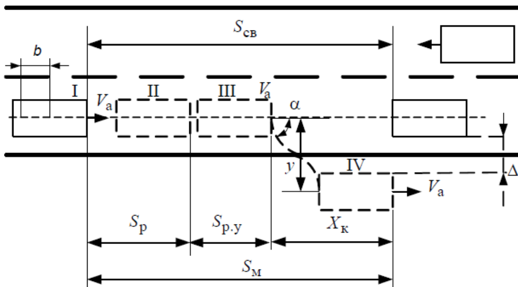
Рис. 6. – Схема объезда препятствия
