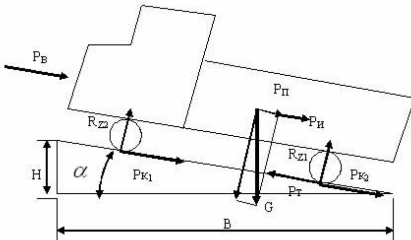
Рис.7. Силы действующие на транспортное средство
