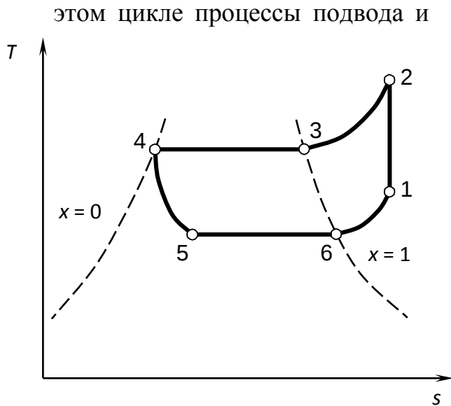
Рис. 5.3. Цикл теплового насоса, работающего на перегретом паре
