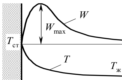
Рис. 8.2. Изменение температуры и скорости жидкости
