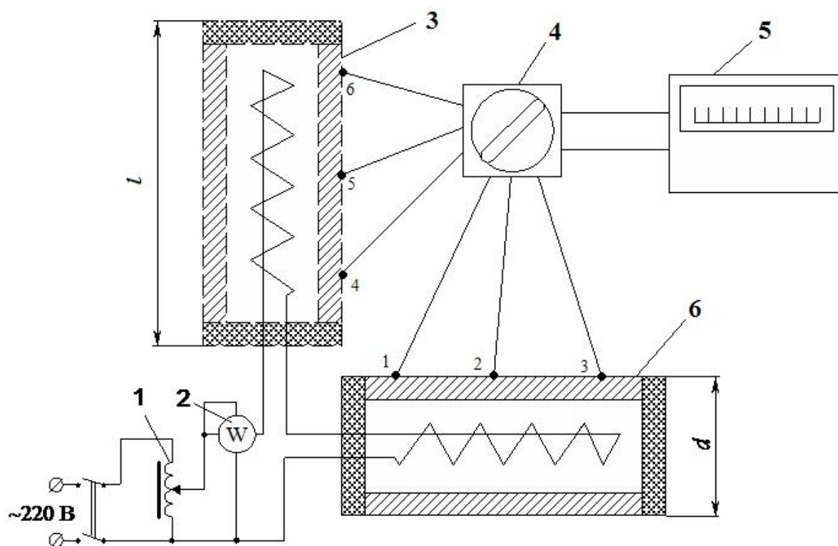
Рис. 8.4. Схема экспериментальной установки
