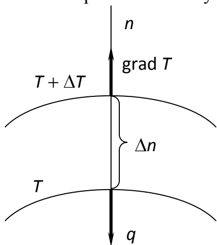
Рис. 6.1. Схема к определению градиента температуры
