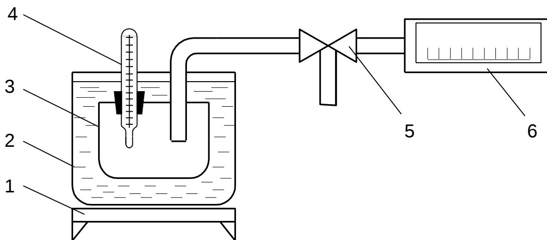
Рис. 1.2. Схема экспериментальной установки
