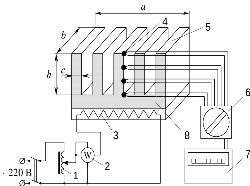
Рис. 8.2. Схема экспериментальной установки
