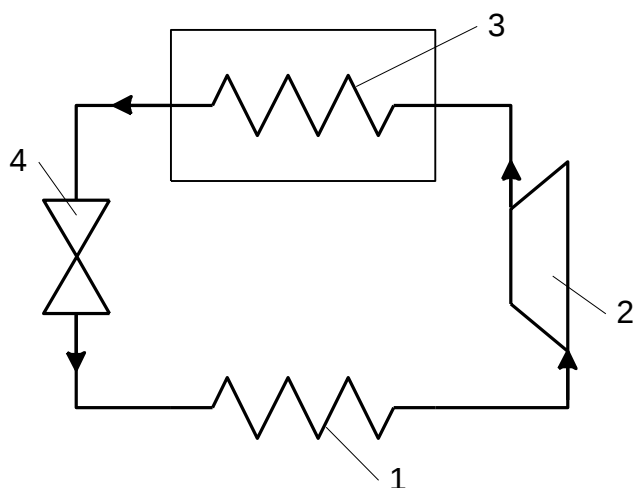
Рис. 5.1. Схема теплового насоса
