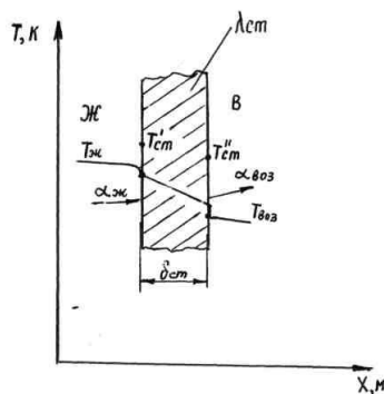
Рис.10.1. Схема процесса теплопередачи
