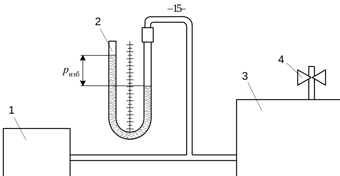
Рис. 2.2. Схема экспериментальной установки
