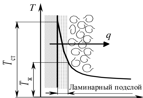
Рис. 8.1. Ламинарный пристеночный слой
