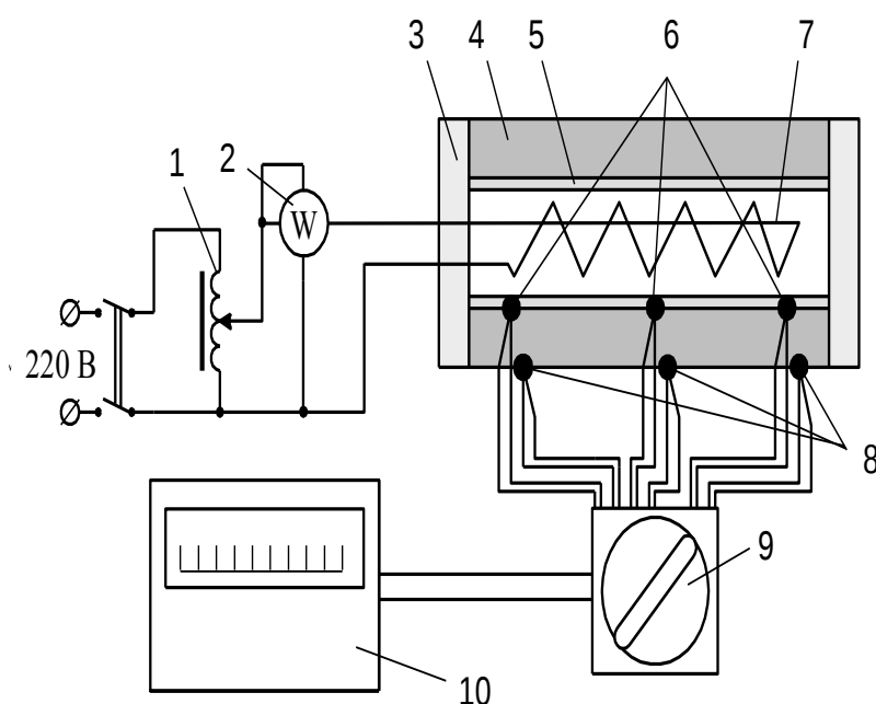
Рис. 6.2. Схема экспериментальной установки
