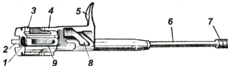
Рис. 10. Затворная рама со штоком
