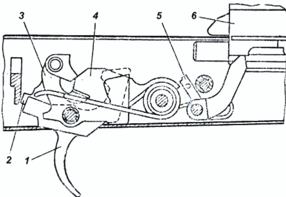
Рис. 18. Положение частей ударно-спускового механизма после выстрела при переводчике, установленном на одиночный огонь
