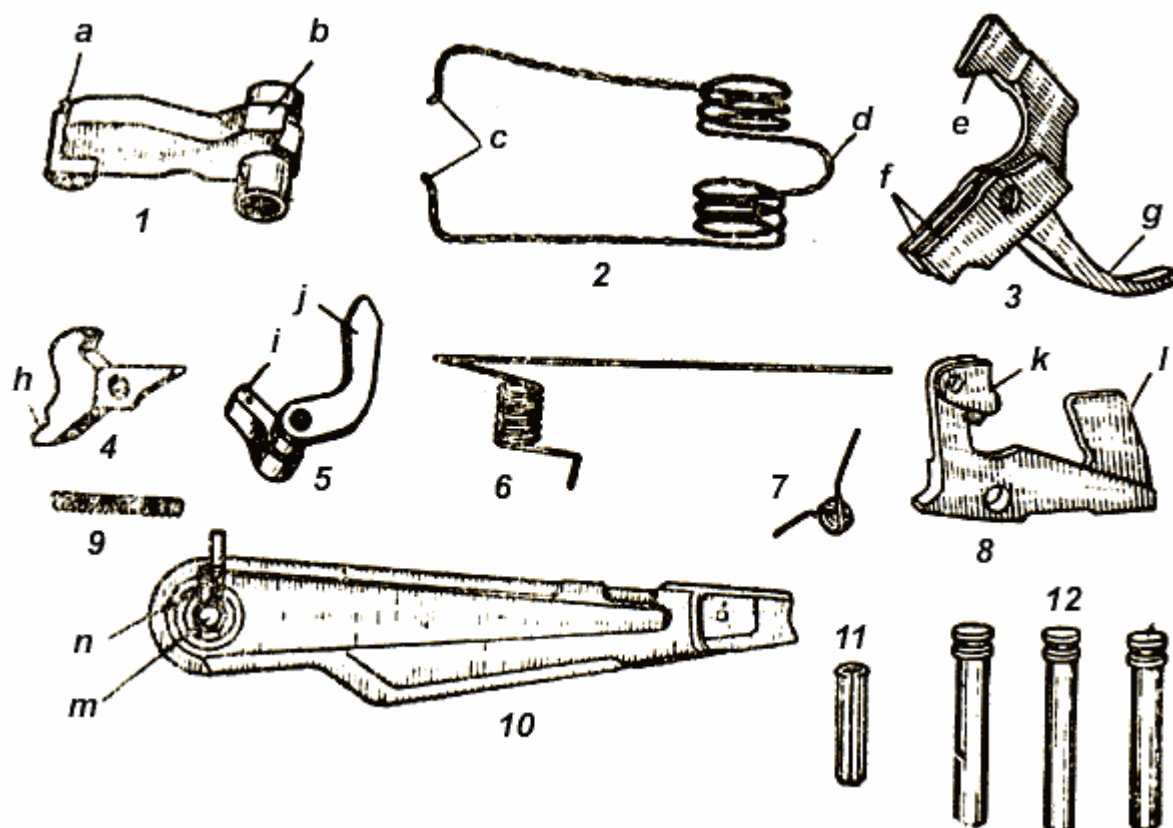
Рис. 14. Ударно-спусковой механизм
