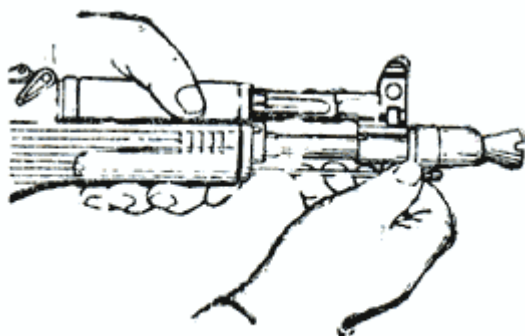
Рис. 25. Отделение шомпола
