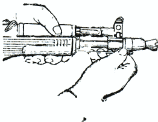
Рис. 25. Отделение шомпола
