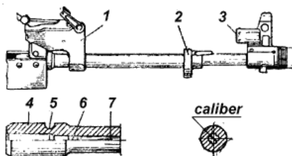
Рис. 3. Ствол
