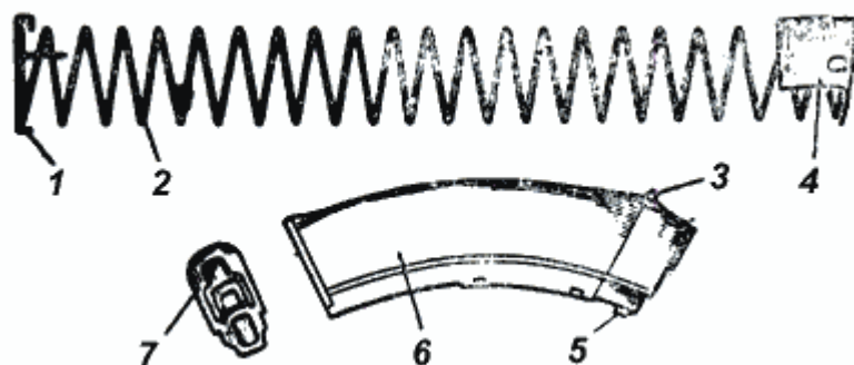
Рис. 19. Магази́н
