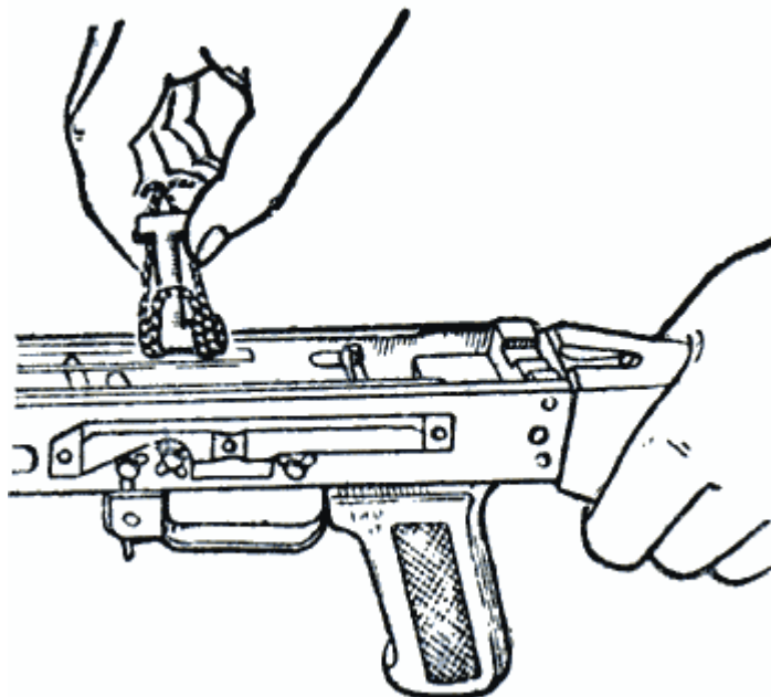
Рис. 37. Извлечение курка из ствольной коробки
