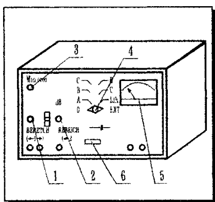
Рис.3. Общий вид измерителя шума
