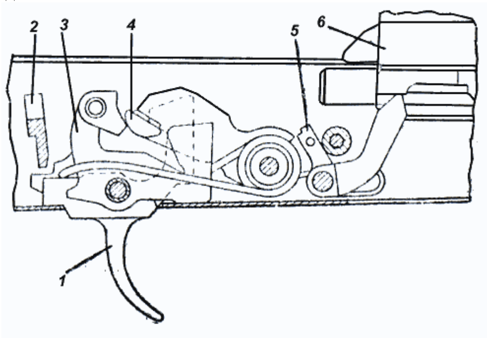
Рис. 17. Положение частей ударно-спускового механизма перед выстрелом
