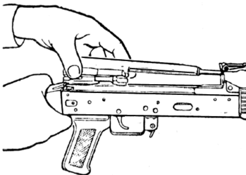
Рис. 28. Отделение затворной рамы с затвором
