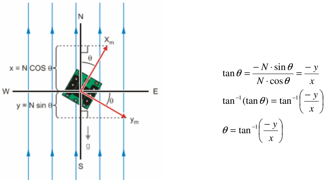
Рис. 4.2 Геометрические соотношения
