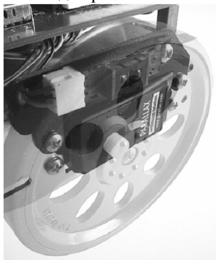
Рис. 5.1 Установленный энкодер
