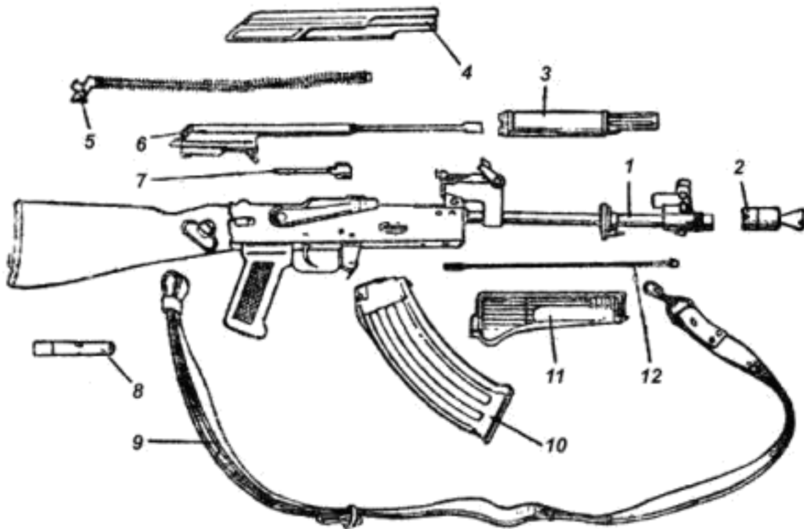
Рис. 2. Основные части и механизмы автомата и его принадлежности
