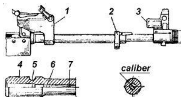
Рис. 3. Ствол
