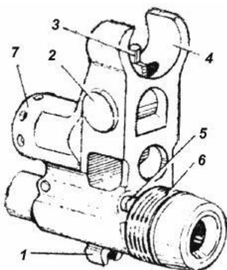
Рис. 5. Колодка мушки
