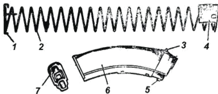
Рис. 19. Магази́н
