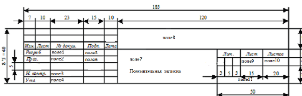
Рисунок 2-Основная надпись для текстовых документов (форма 2)
