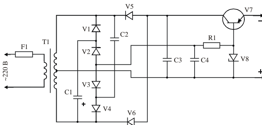
Рисунок 6.4- Нумерация элементов на схеме стабилизированного источника постоянного напряжения
