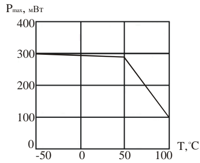
Рисунок 5.6- Зависимость допустимой рассеиваемой мощности на стабилитронах КС156А и КС168А от температуры.
