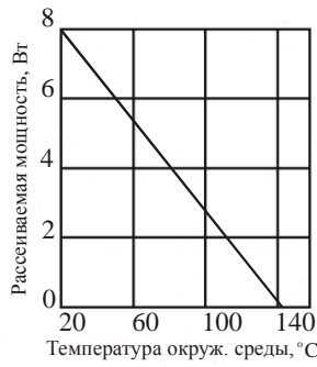
Рисунок 5.5- Тепловая характеристика радиатора для транзистора с предельной температурой перехода 125^{\circ}\text{C} .
