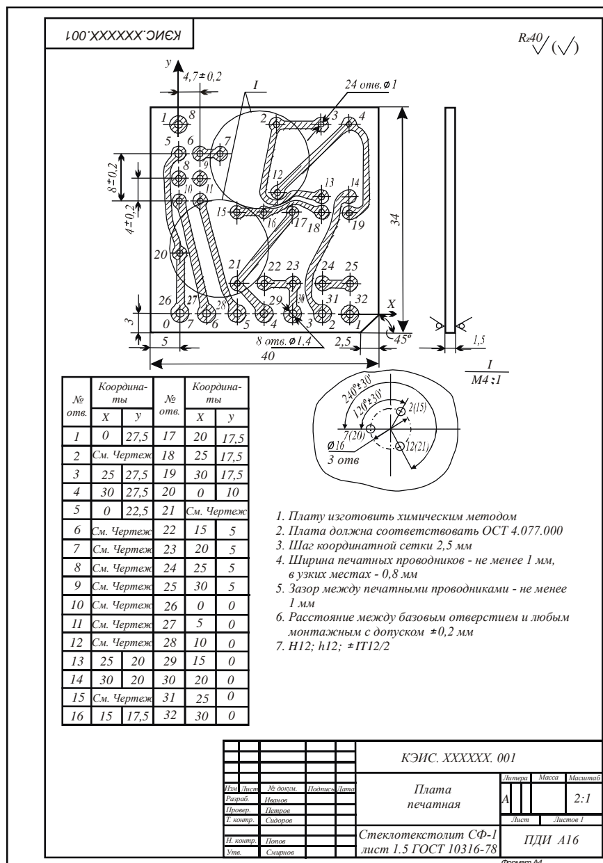
Рисунок 7.6 - Чертеж печатной платы с проводниками произвольной формы
