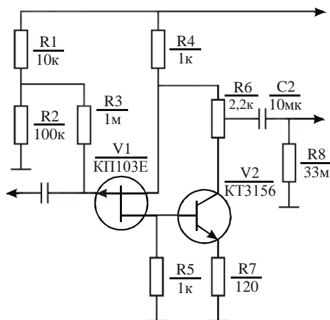
Рисунок 6.5- Пример записи номиналов резисторов, конденсаторов и маркировки транзисторов на схеме усилителя
