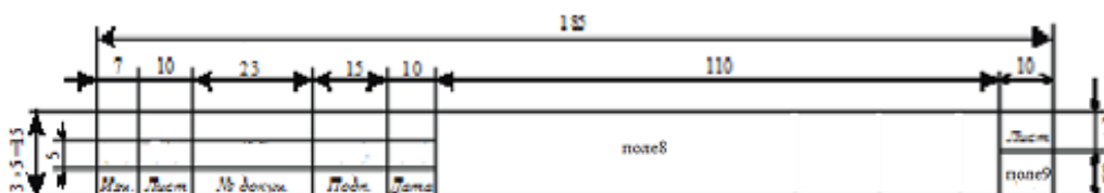
Рисунок 3-Основная надпись для остальных страниц чертежей и текстовых документов (форма 2а)
