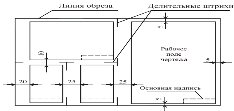
Рисунок 6.1- Выделение форматов и нанесение рамок на бумажном листе
