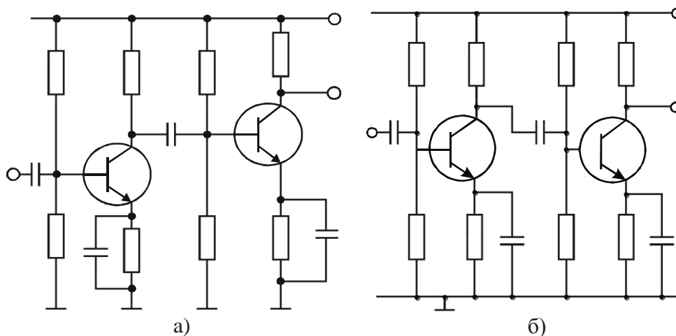
Рисунок 6.3- Элементы схемы не выровнены по горизонтали, изображение каскадов разное, ненужные повороты линий связи (а), элементы схемы размещены и соединены рационально (б).
