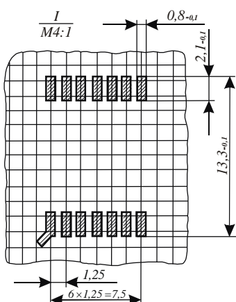
Рисунок 7.4- Изображение контактной группы
