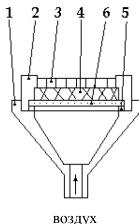
Рис. 4 Схема ячейки для испытания мембран:
