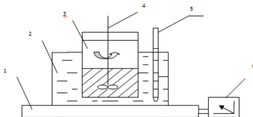
Рис. 1. Установка для приготовления растворов ПА-6 - МК - Н 2 О
