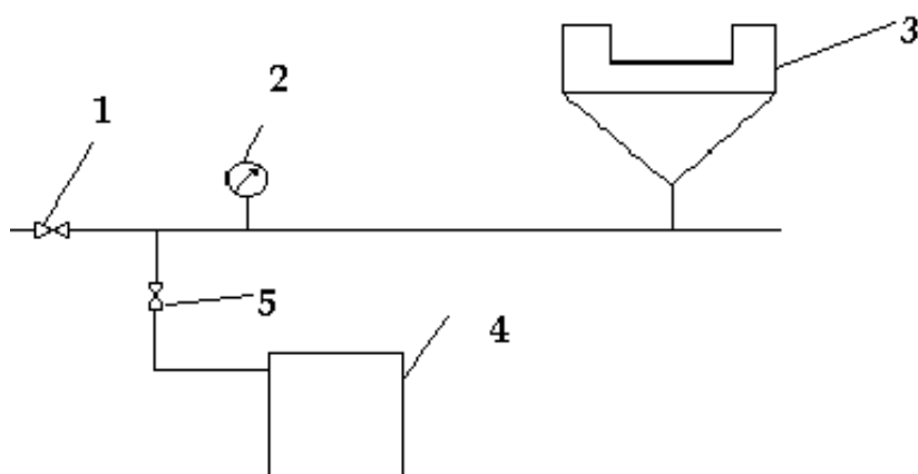
Рис. 3. Схема установки для определения точки пузырька
