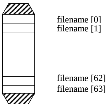
Рис. 13. Трактовка символьной строки как массива типа char
