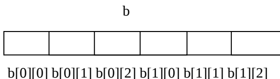
Рис. 11. Размещение двумерного массива в памяти
