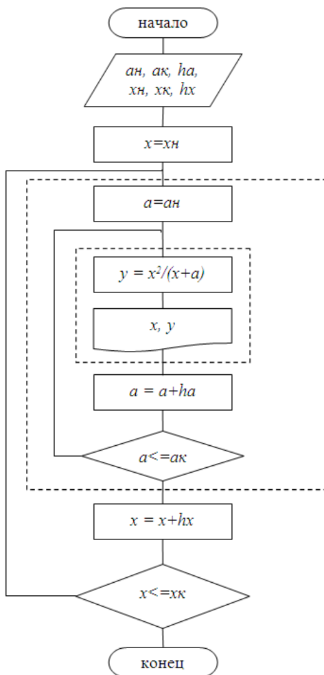
Рис. 8. Блок-схема алгоритма со вложенным циклом
