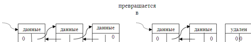
Рис. 20. Удаление элемента двусвязного списка
