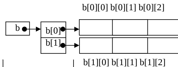
Рис. 11. Размещение двумерного массива в памяти
