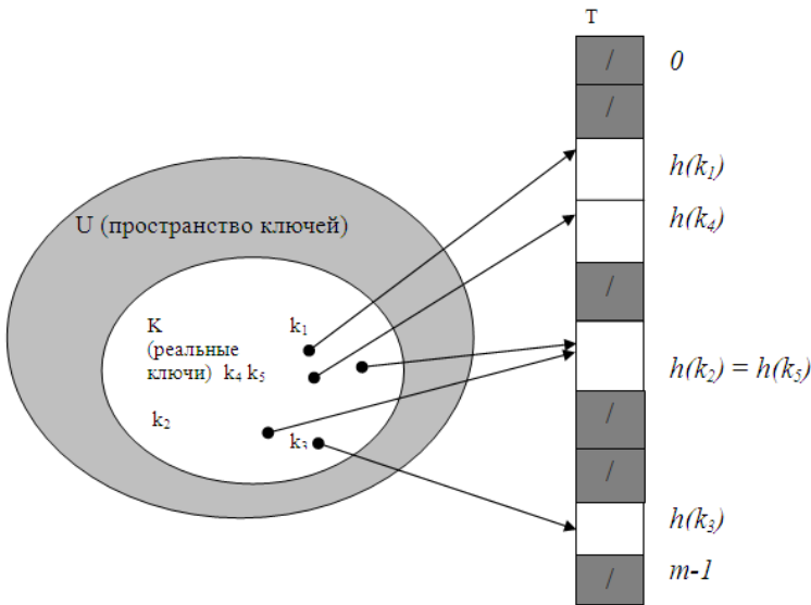
Рис. 24. Использование хеш-функции h для отображения ключей в ячейки хеш-таблицы
