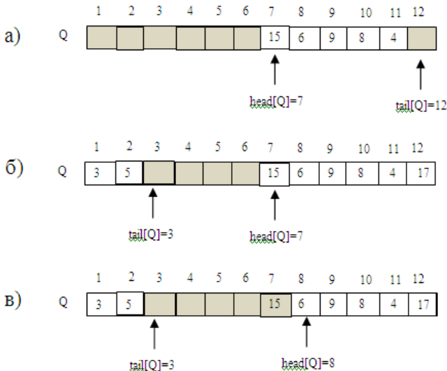
Рис. 22. Очередь, реализованная с помощью массива Q[1..12]
