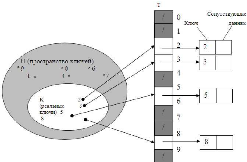
Рис. 23. Реализация динамического множества с использованием таблицы с прямой адресацией
