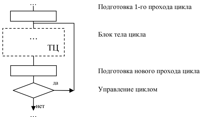
Рис. 2. Схема цикла с постусловием
