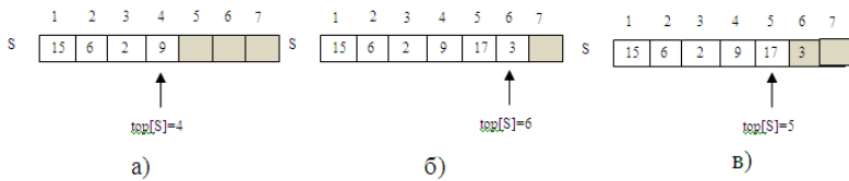
Рис. 21. Реализация стека S в виде массива
