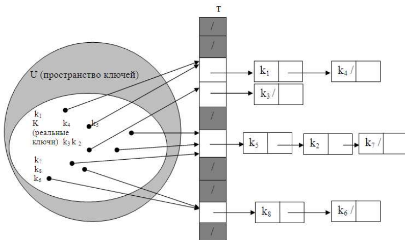
Рис. 25. Разрешение коллизий при помощи цепочек
