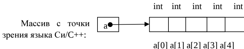
Рис. 10. Массив с точки зрения языка Си/C++
