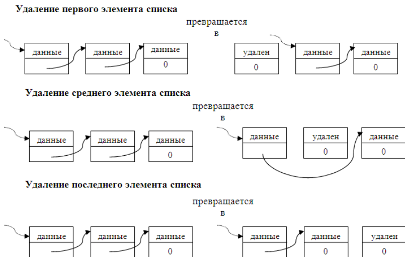
Рис. 17. Удаление элемента из односвязного списка
