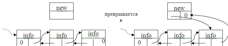
Рис. 19. Добавление элемента в двусвязный список
