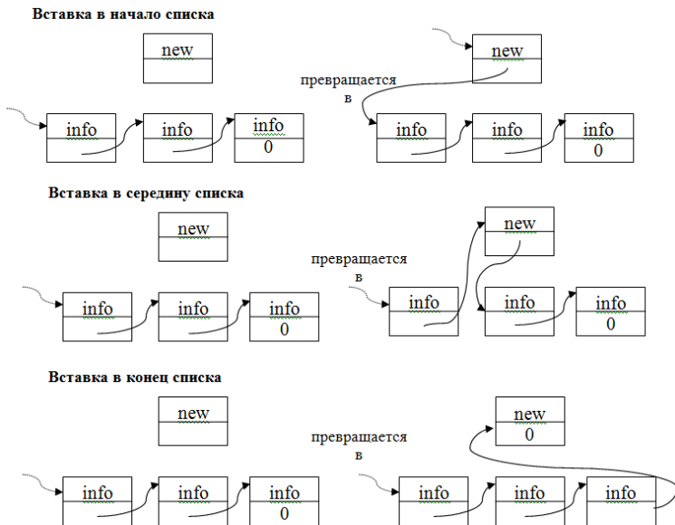
Рис. 16. Вставка нового элемента в односвязный список
