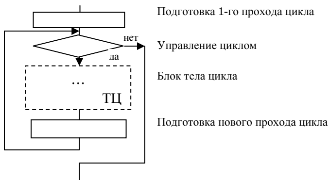
Рис. 1. Схема цикла с предусловием
