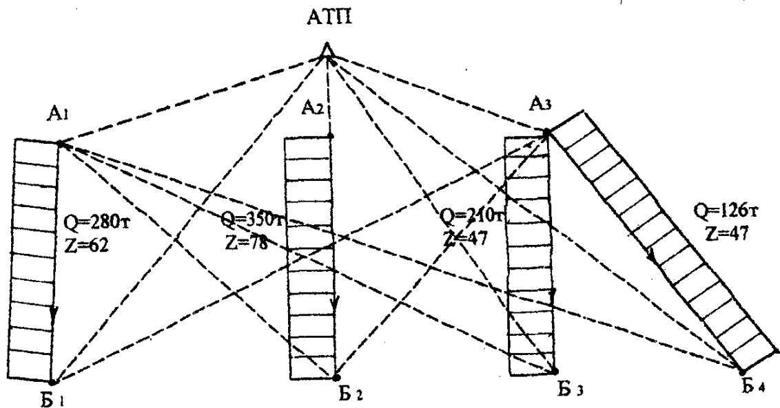
Рис. 7 Эпюра грузопотоков
