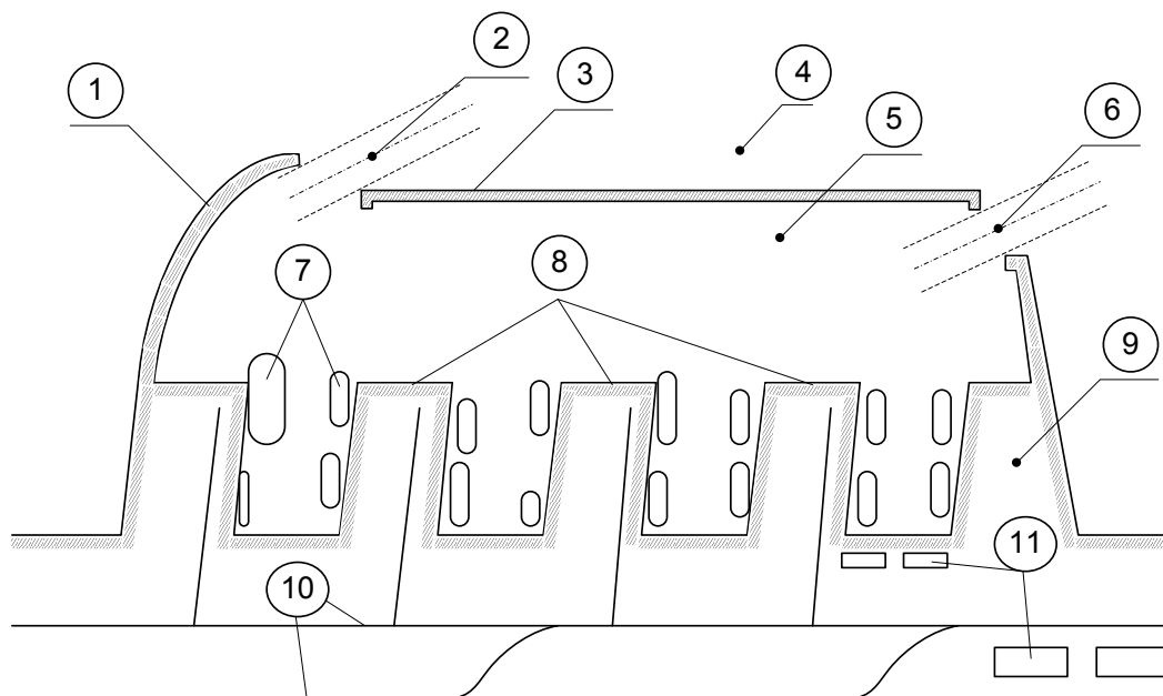
Рисунок 7.2 – Основные элементы порта: 1 – мол; 2 – ось выхода из порта; 3 – волнолом; 4 – внешний рейд; 5 – внутренний рейд; 6 – ось входа в порт; 7 – плавсредства; 8 – широкие причалы; 9 – пассажирская площадка; 10 – железнодорожные пути; 11 – склады
