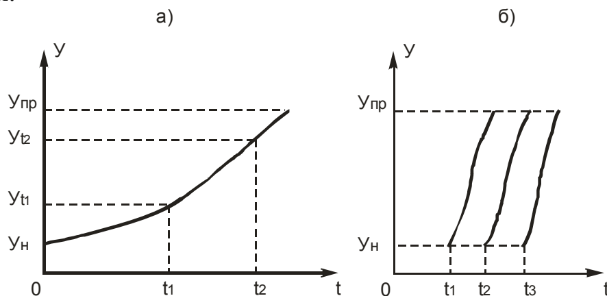
Рис.1.3. Изменение параметра технического состояния U по наработке t при постепенных (а) и внезапных (б) отказах. U_H ; U_{пр} – начальное и предельное значения параметров
