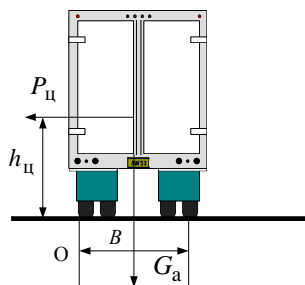
Рис. 15. Действие в поперечной плоскости моментов от сил P_{\text{ц}} и
