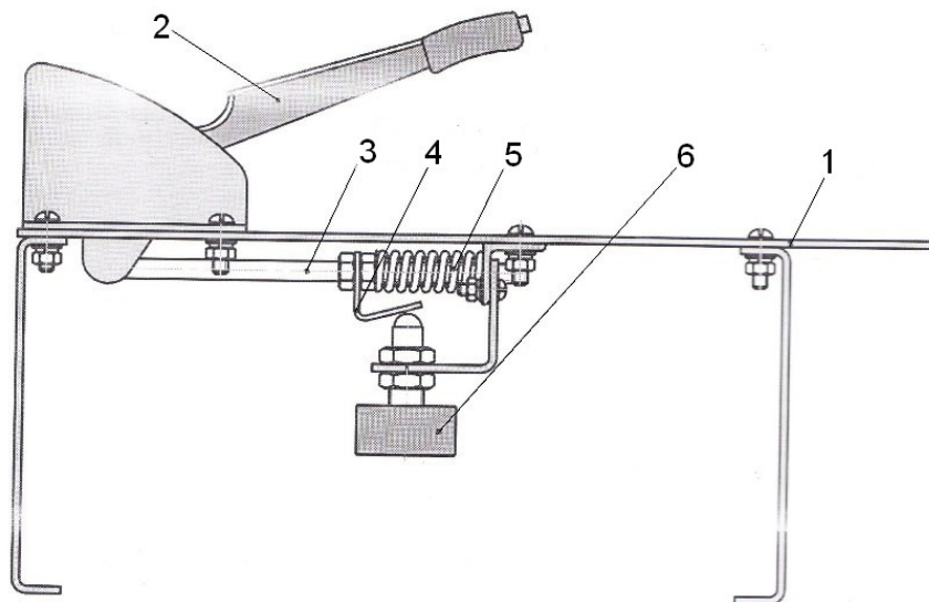
Рис. 5. Имитатор стояночной тормозной системы: 1 – корпус, 2 – рычаг стояночной тормозной системы, 3 – толкатель, 4 – нажимная планка, 5 – пружина имитации усилия, 6 – электрический датчик (выключатель)
