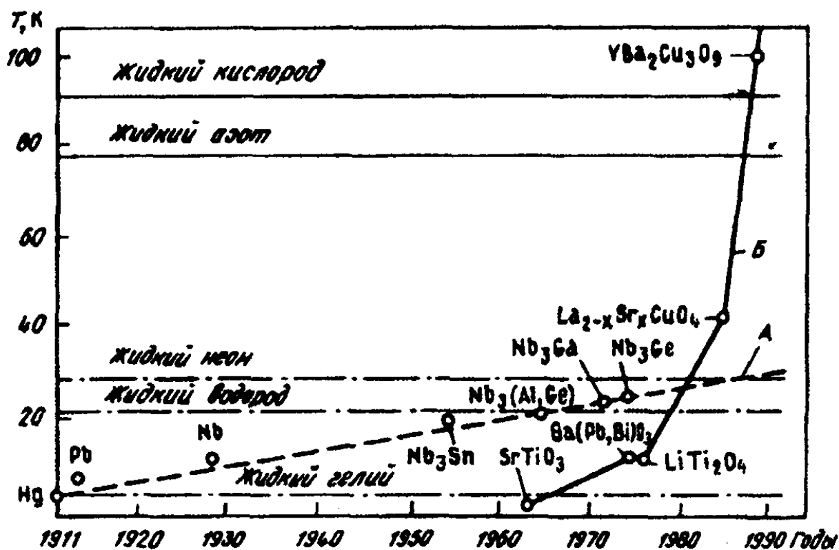
Рис.6. Динамика разработок сверхпроводников: А — металлические материалы; Б — керамика
