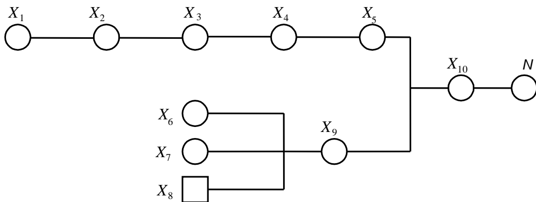
Рис. 6. Дерево причин аварии автомобиля-тягача:
