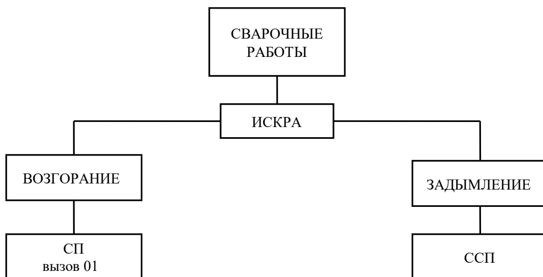
Рис. 7. Дерево событий при выполнении сварочных работ: а – принципиальная схема; б – диаграмма событий
