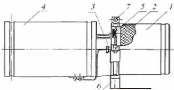
Рис. 2.5. Принципиальная схема аэрозольного генератора: 1 – корпус; 2 – аэрозолеобразующий состав; 3 – узел запуска; 4 – инжектор; 5 – сопловое отверстие; 6 – кронштейн.
