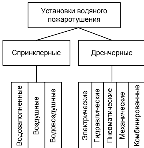
Рис. 2.4. Классификация установок водяного пожаротушения
