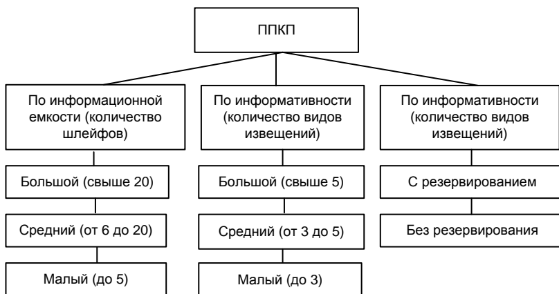
Рис. 2.11. Классификация ППКП
