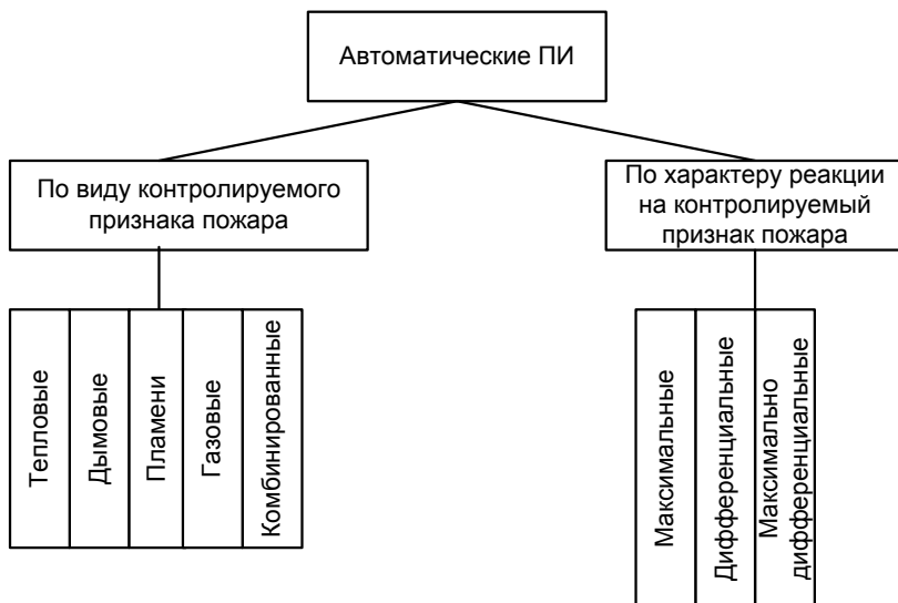
Рис. 2.10. Классификация автоматических пожарных извещателей.
