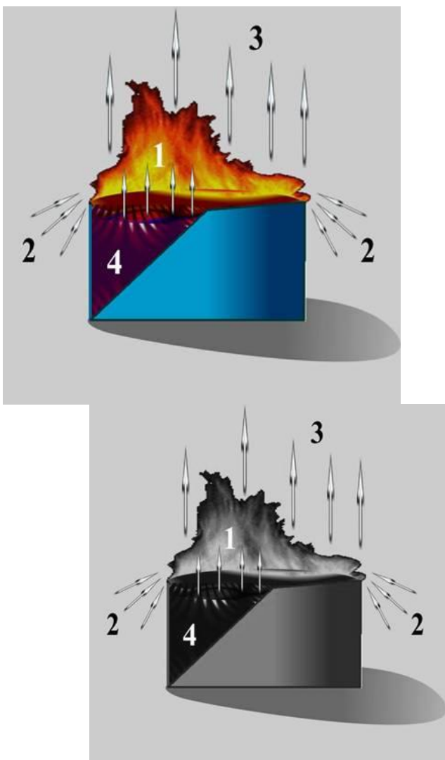
Рис. 1.1. Схема диффузионного горения жидкости 1 – пары горючей жидкости; 2 – воздух, подсосываемый в зону горения по законам газовой конвекции; 3 – продукты горения; 4 – жидкость в резервуаре
