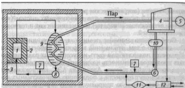
Рис. 2.37. Принципиальная технологическая схема АЭС:
