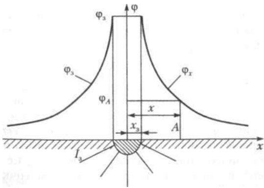
Рис. 2.32. Растекание тока в грунте
