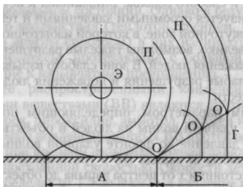
Рис. 2.41. Волнообразование при воздушном взрыве в приземной зоне:
