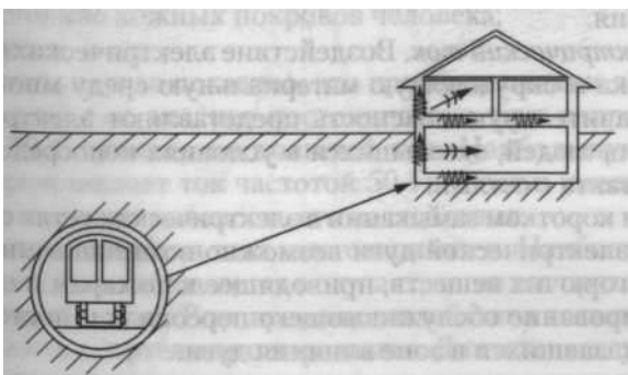
Рис- 2.31. Распространение вибраций от поезда метрополитена по грунту
