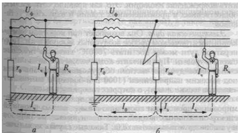
Рис. 2.36. Прикосновение человека к фазному проводу трехфазной четырехпроводной сети с заземленной нейтралью:
