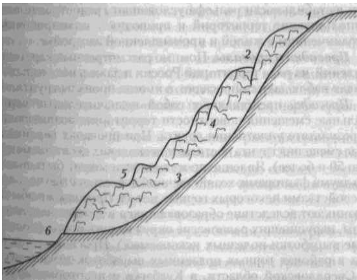
Рис. 2.42. Принципиальная схема оползневого склона:
