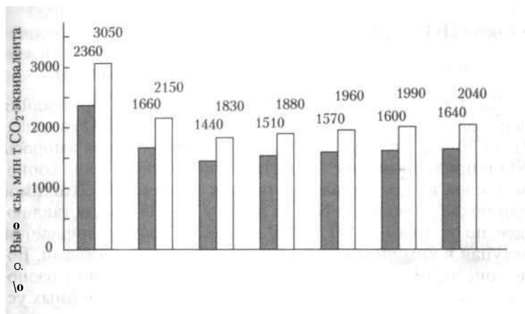
Рис. 2.26. Техногенные выбросы парниковых газов (CO 2 — эквивалент в год): 1 — CO 2 ; 2 — все парниковые газы
