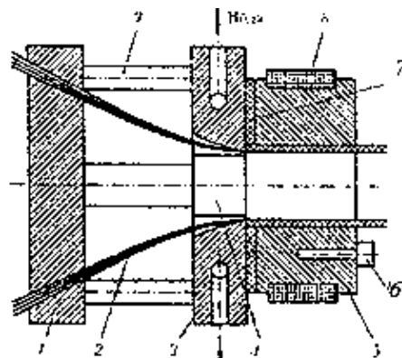
Рис. 2.28. Формующая матрица пултрузионного агрегата
