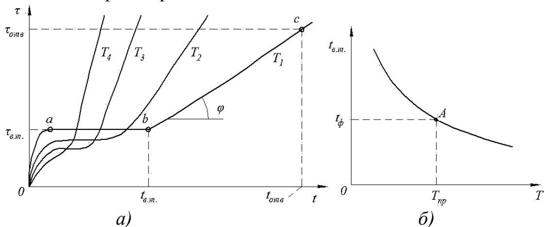
Рис. 2.6. Зависимость напряжения сдвига от времени пребывания пресс-материала в пластометре при различных температурах T_1 < T_4 , (а) и продолжительности вязкотекучего состояния от температуры (б)
