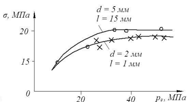
Рис. 2.8. Зависимость разрушающего напряжения при растяжении от давления в форме для материала Вх4-080-34 при различных диаметре d и длине l литника
