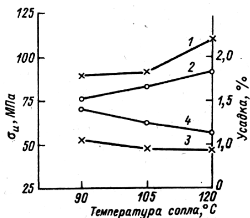
Рис. 2.20. Зависимость разрушающего напряжения при изгибе \sigma_{и} (1, 2) и усадки (3, 4) от температуры сопла литьевого цилиндра: 1, 3 – веерный литник; 2, 4 – долевой литник
