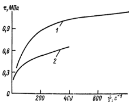
Рис. 2.1. Зависимость напряжения сдвига от скорости сдвига для пресс-материалов: 1 – пресс-порошок Эб-014-30, 150 °C; 2 – стекловолокно АГ-4В, 140 °C
