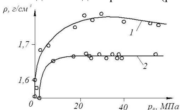
Рис. 2.7. Зависимость плотности изделия от давления в форме для различных пресс-материалов: 1 — Вх4-080-34; 2 — АГ-4
