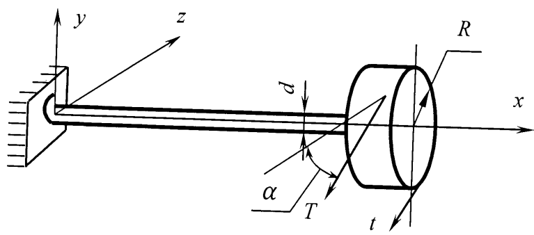
Рис. 10. К расчету вала на изгиб с кручением
