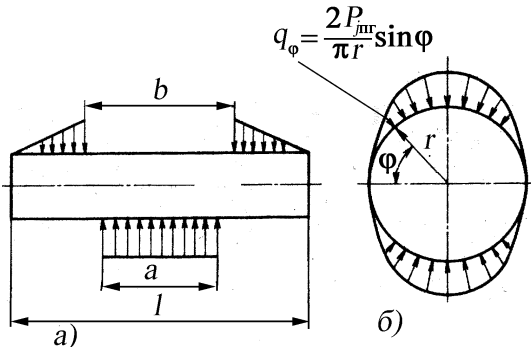
Рис. 3. Расчетные схемы нагружения поршневого пальца от сил инерции P_{jn\sigma} : а – при расчете на изгиб и срез; б – при расчете на овализацию
