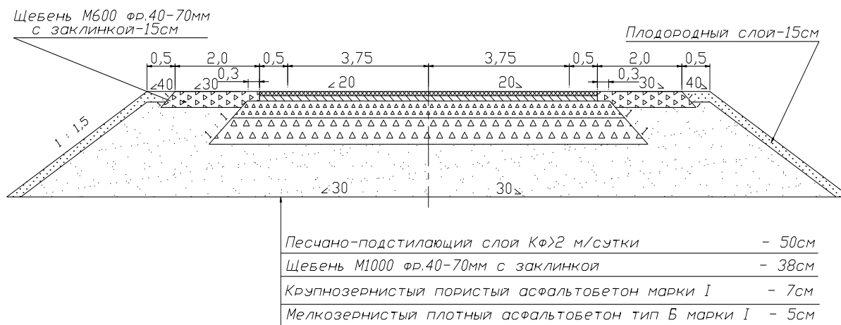
Рис. 7. Конструкция дорожной одежды
