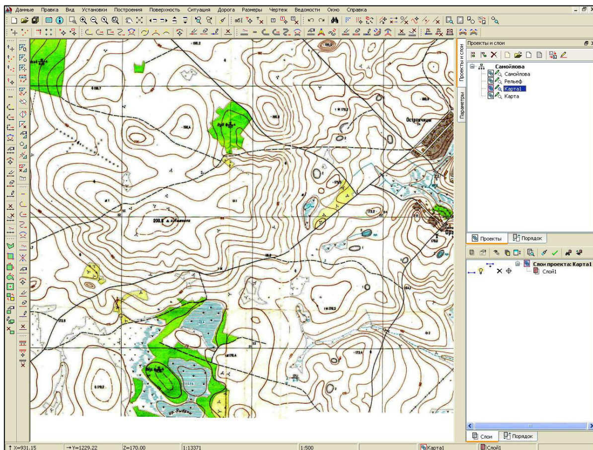
Рис. 1. Интерфейс окна План системы CREDO Дороги
