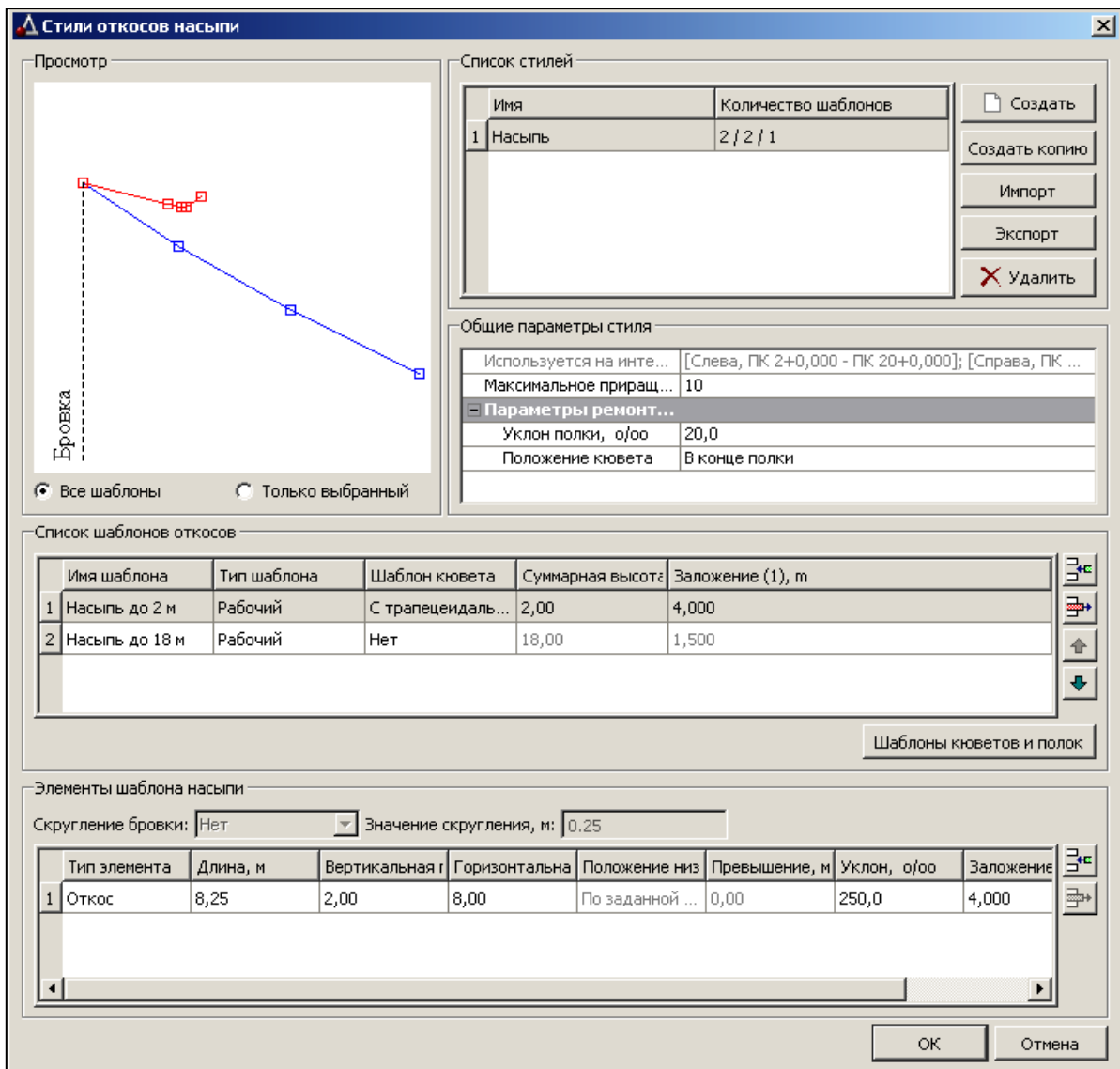
Рис. 6. Вкладка Стили откосов насыпи
