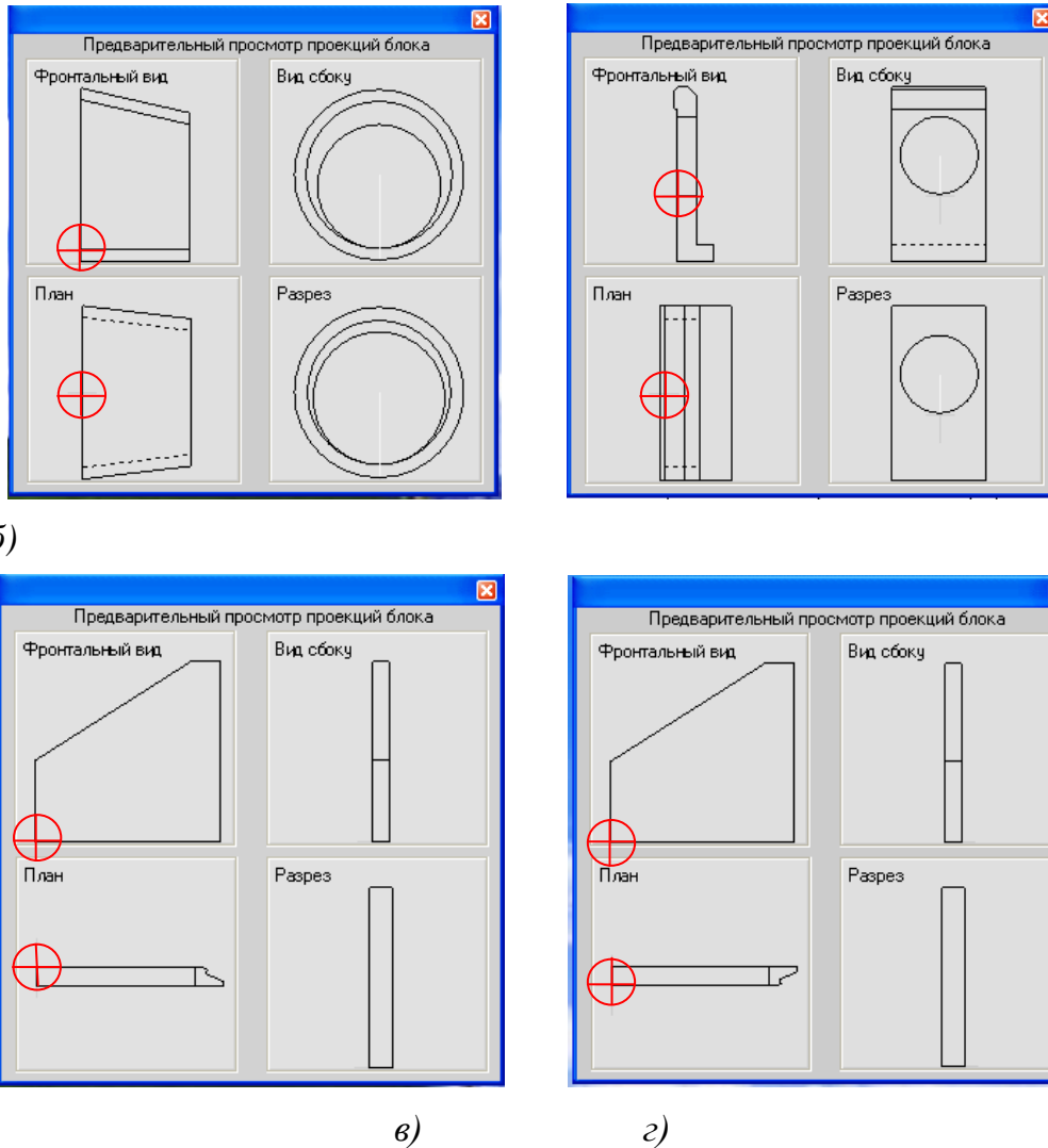
Рис. 23. Точки вставки: а – коническое звено на входе; б – порталная стенка; в – правая откосная стенка; г – левая откосная стенка
