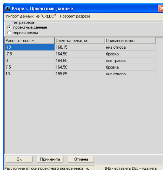
Рис. 17. Данные для поперечного профиля автодороги: а – черная земля; б – проектные данные
