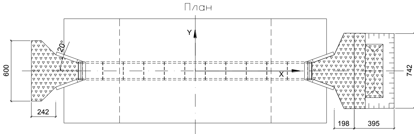
Рис. 13. Чертеж водопропускной трубы
