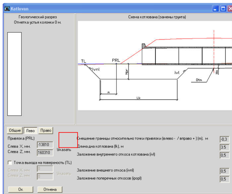
Рис. 26. Размеры котлована: a – общие по оси трубы; b –слева (справа) под оголовок
