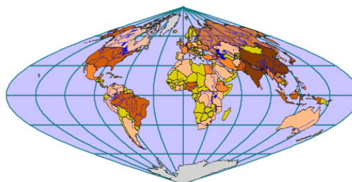
Проекция Синусоидальная (Sinusoidal), тип - псевдо- цилиндрическая (Pseudo-Cylindrical)
