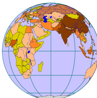
Проекция Ортогональная (Orthographic), тип - планарная (Planar)
