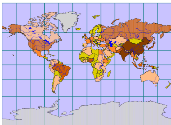
Проекция Миллера (Miller Cylindrical), тип - цилиндрическая (Cylindrical)
