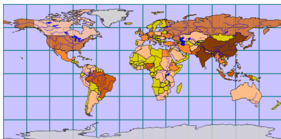
Географическая проекция (Geographic), тип - сферическая (Spherical)
