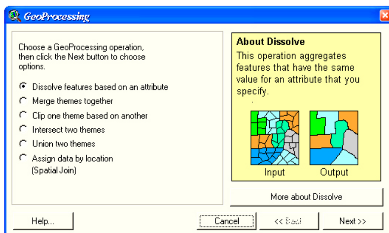
Рис. 1. Модуль Geoprocessing
