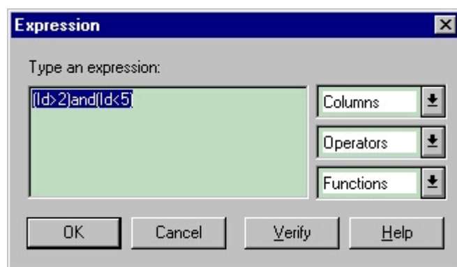
Рис. 2. Диалог Expression
