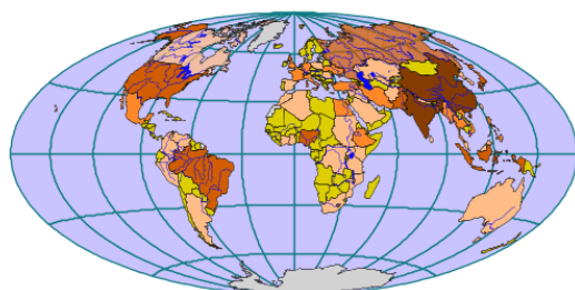
Проекция Хаммера-Аитоффа (Hammer-Aitoff), тип - модифицированная планарная (Modified Planar)
