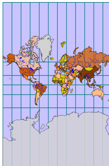
Проекция Меркатора (Mercator), тип - цилиндрическая (Cylindrical)
