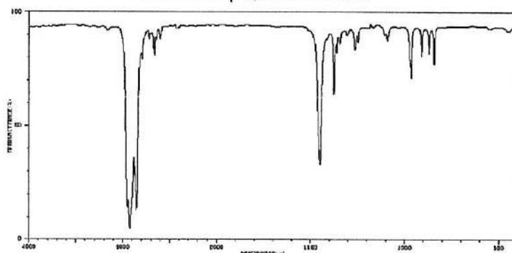
ИК-спектр циклогексана
