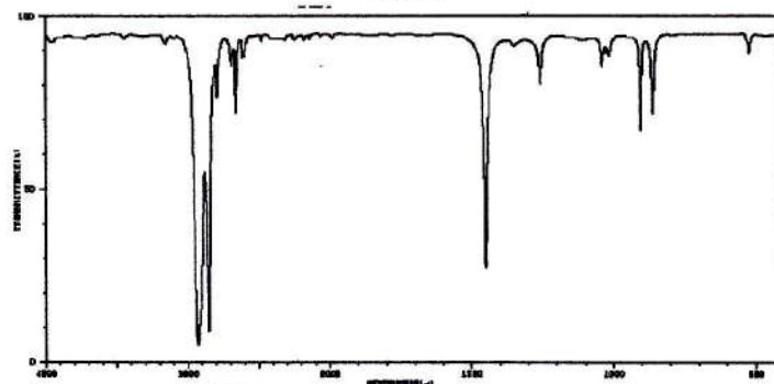
ИК-спектр циклогексана
