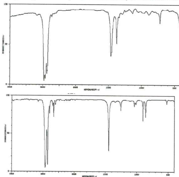
ИК-спектр циклогексана
