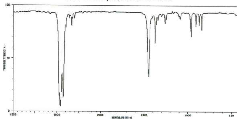
ИК-спектр метилциклогексана
