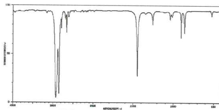
ИК-спектр циклогексана
