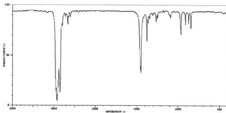
ИК-спектр метилциклогексана
