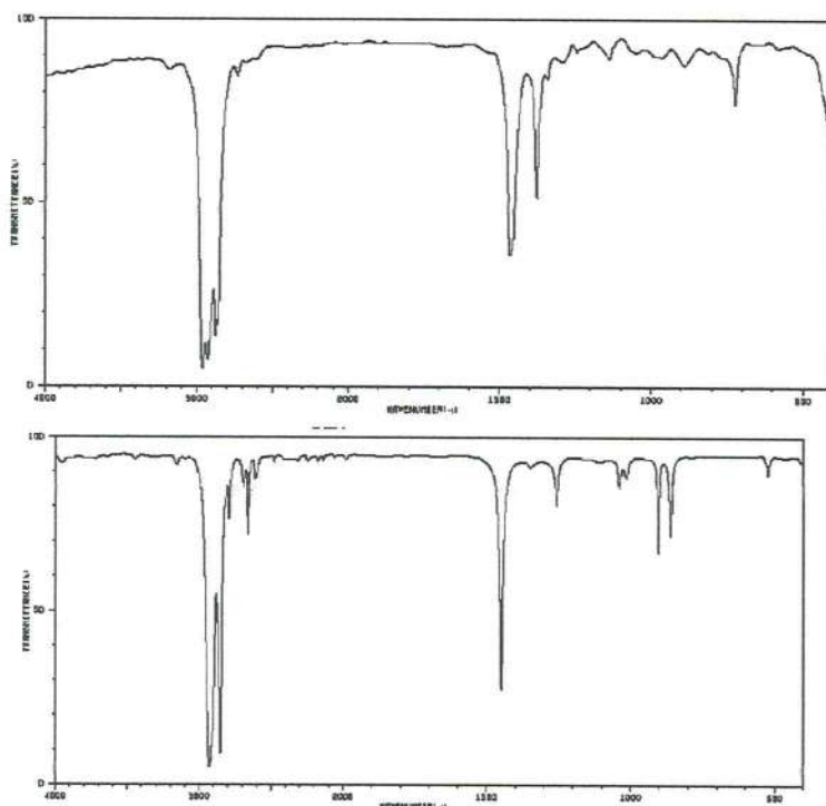
ИК-спектр циклогексана
