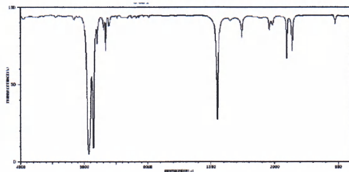
ИК-спектр циклогексана
