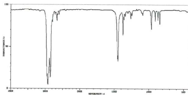
ИК-спектр метилциклогексана
