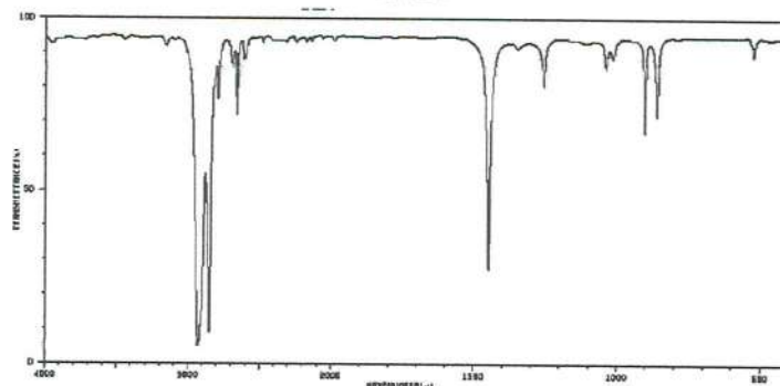
ИК-спектр циклогексана
