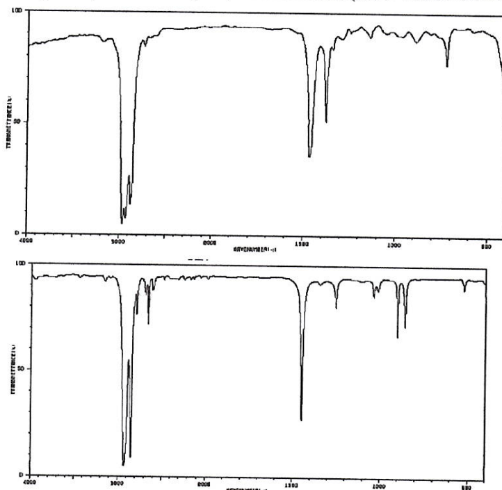
ИК-спектр циклогексана
