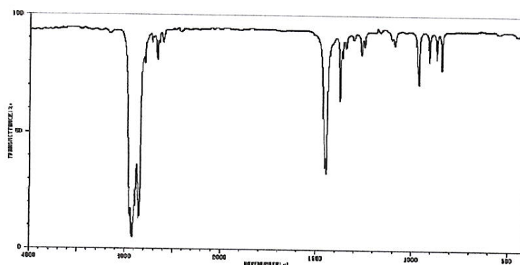
ИК-спектр метилциклогексана
