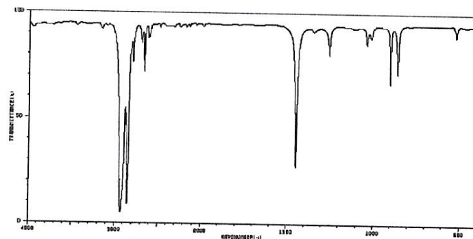
ИК-спектр циклогексана
