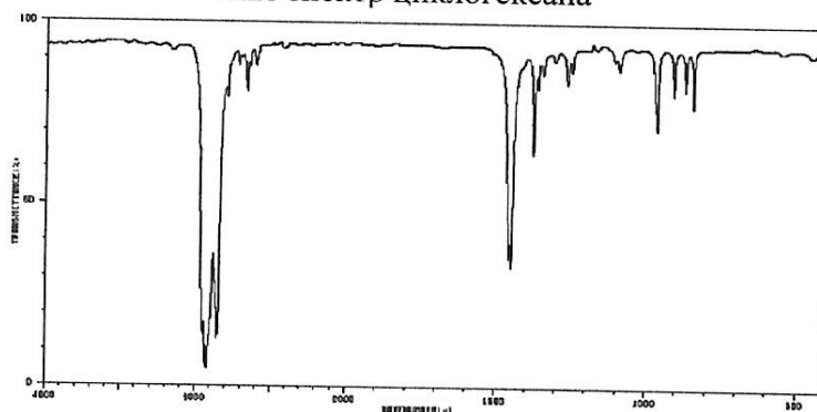
ИК-спектр метилциклогексана
